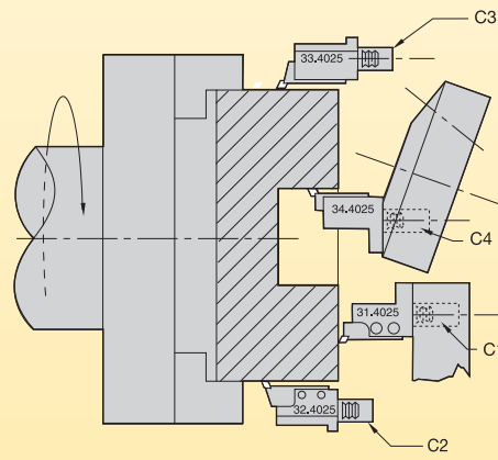
右勝手（反時計回り）のスピンドル回転
