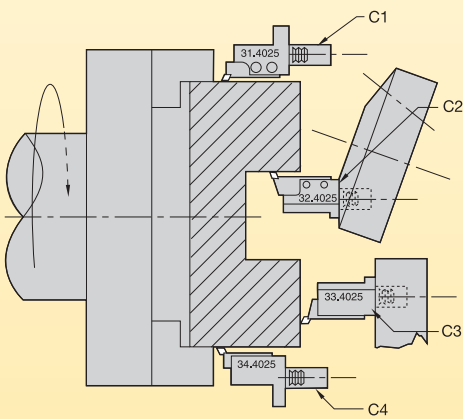
左勝手（時計回り）のスピンドル回転
